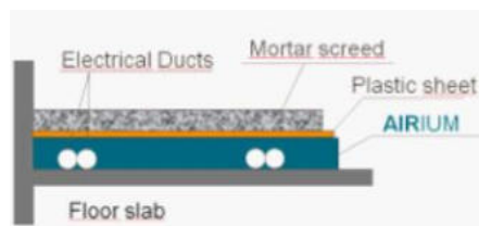
Abbildung 4: Schematische Darstellung der Ausgleichsschüttung-Anwendung von Airium – Quelle: Holcim Technology Ltd
